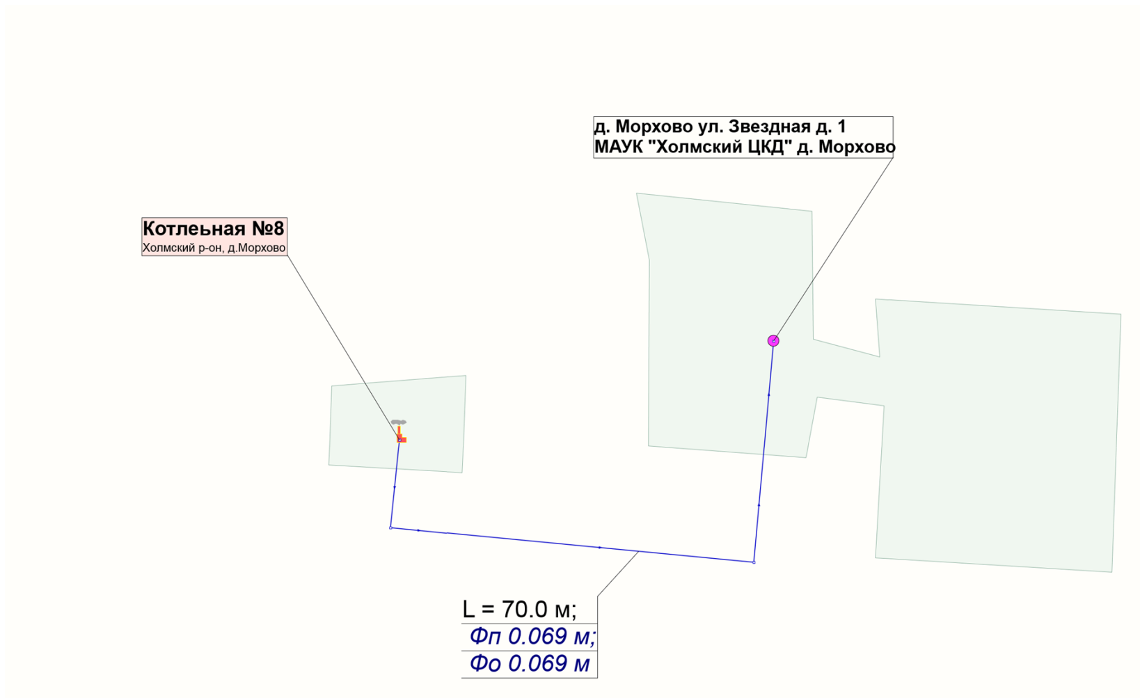
Рисунок 1.1 Схема тепловых сетей котельной №8, д. Морхово
